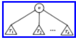
Fig. 3.4. Tree T .
