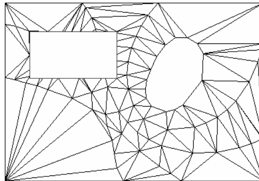
Figure 14.19 - Le maillage troué en plan
