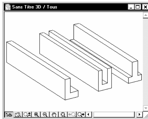
Figure 11.10 - Intersection de poutre en volume
