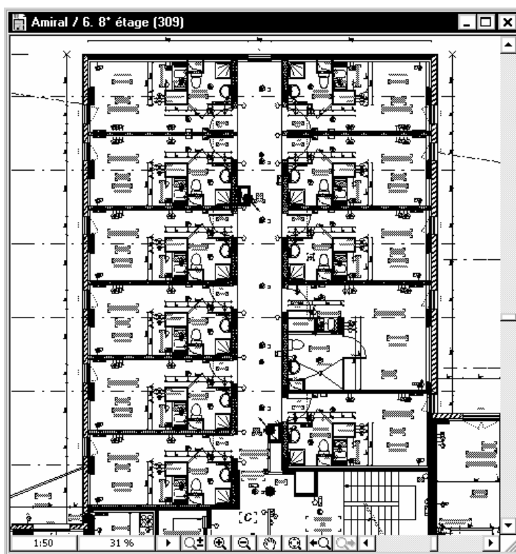
Figure 41.3 - Exemple d'un projet dont les niveaux sont constitués de modules.
