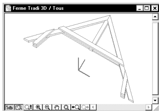
Figure 40.11 - La ferme visualisée en 3D
