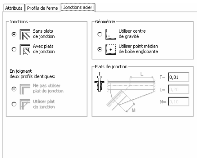
Figure 38.38 - La palette des options TrussMaker : Onglet jonctions acier
