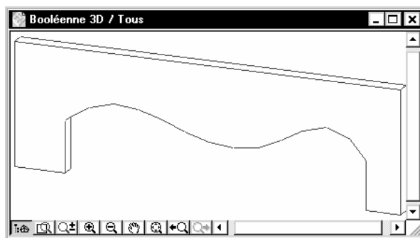
Figure 44.16 - L'élément mur après l'opération élément solide
