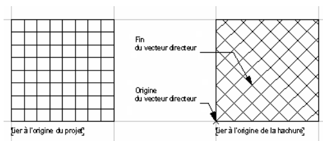
Figure 12.6 - L'origine de la hachure de la dalle
