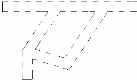
Figure 11.9 - Intersections de poutres en plan
