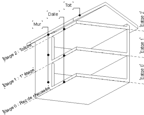
Figure 6.5 - Le principe de gestion des étages
