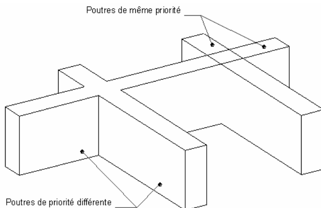
Figure 11.11 - Intersection de poutre en volume par rapport au numéro de priorité
