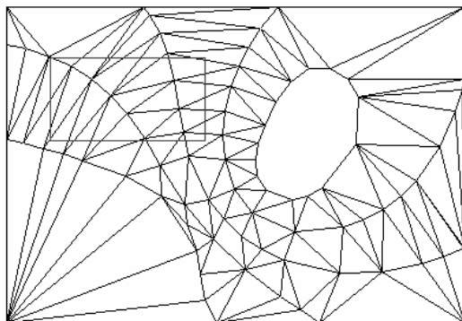
Figure 14.15 - Le maillage terminé en plan
