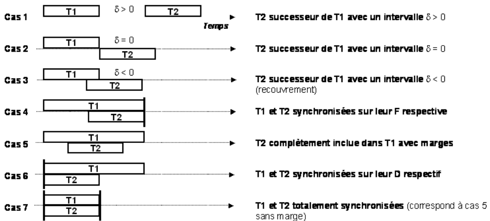
Figure 9.13 - les différents cas d'ordonnancement possibles entre deux tâches
