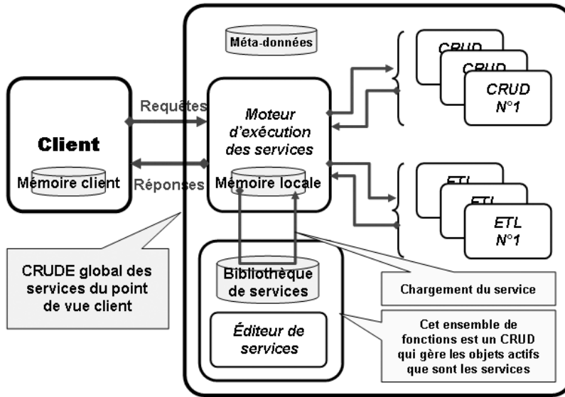
Figure 10.16 - Modèle Client-Services
