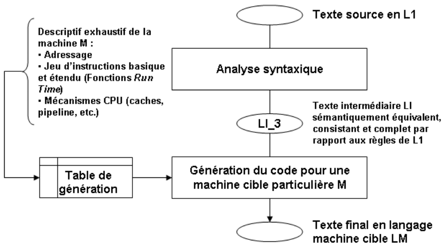
Figure 6.8 - Compilateur complet
