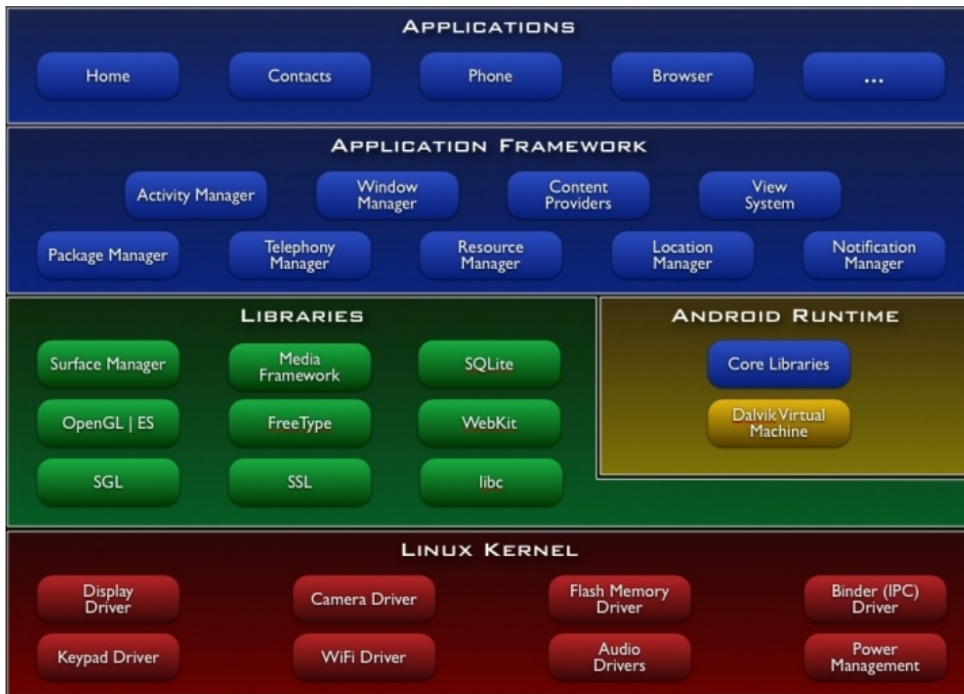
L'architecture d'Android
