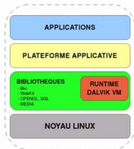
Figure 1-1 L'architecture en couches d'Android
