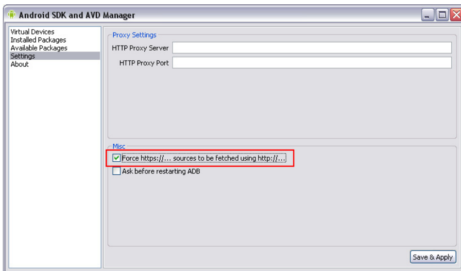
Figure 1-12 Réglage à effectuer pour contourner l'erreur.
