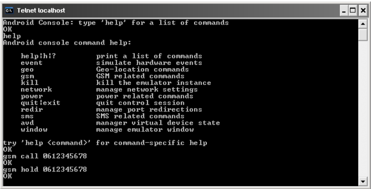
Figure 12-8 Un appel, puis une mise en pause seront obtenus grâce à la commande gsm .
