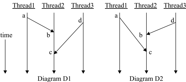
Figure 6.7 Diagrams D1 and D2.
