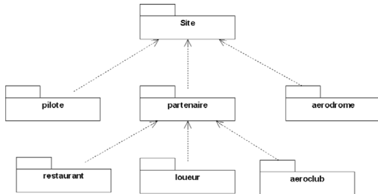
Figure 6-1 La hiérarchie des modèles de notre application
