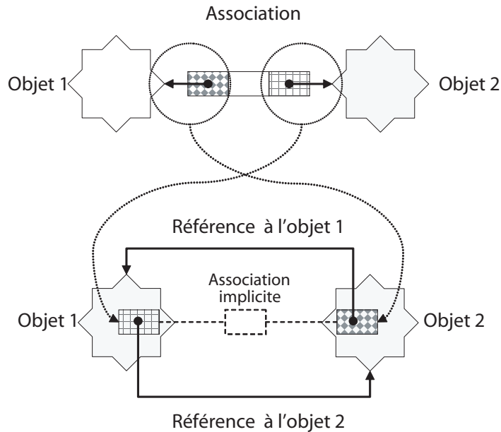
Figure 3-8 Références ayant migré dans les objets
