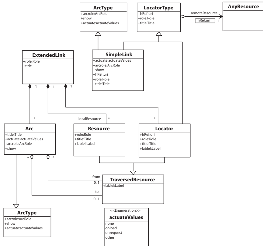
Figure 12-6 Modèle conceptuel de XLink
