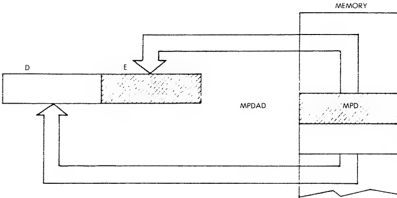
Fig. 3.16: LD DE, (MPDAD)
