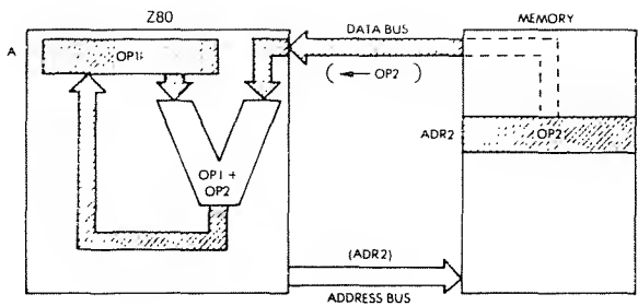
Fig. 3.3: ADD A, (HL)
