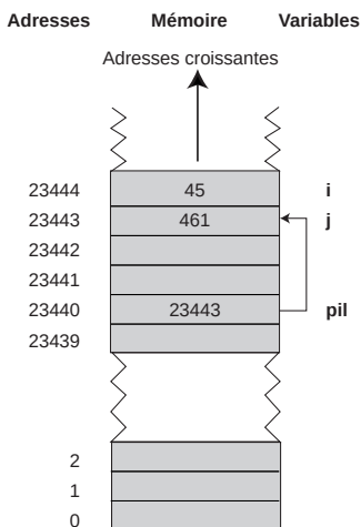
Figure 3.1 : Notions de pointeur et d'adresse
