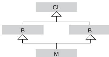
Figure 4.7 : Représentation UML de l'héritage multiple.
