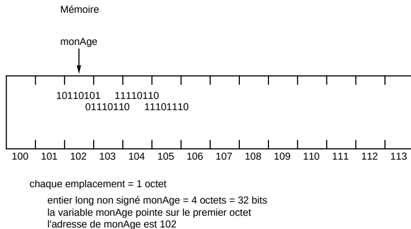
Figure 8.1 Représentation schématique de la variable monAge.
