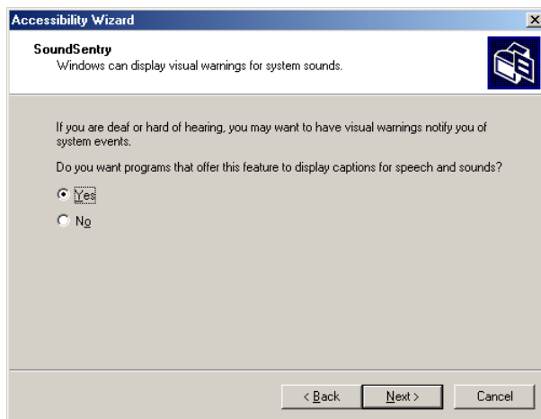
Fig. 24.29 SoundSentry dialog.
