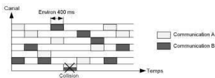
Figure 2.12 — Exemple de partage des ondes avec le FHSS.
