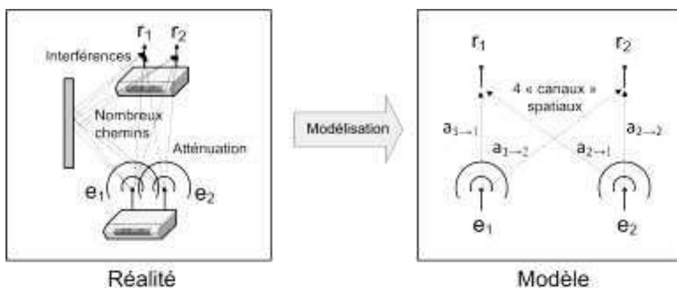
Figure 2.17 — Modèle du multiplexage spatial.
