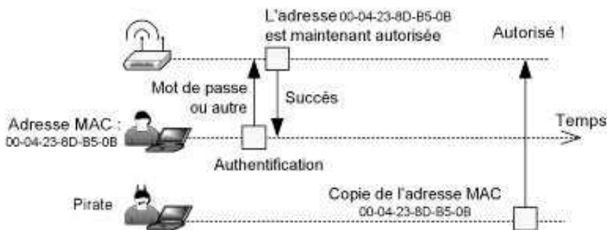
Figure 6.3 — Détournement de session par « spoofing » de l'adresse MAC.
