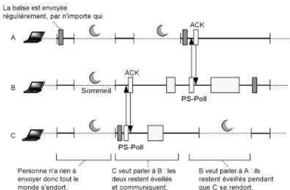
Figure 3.18 — L'économie d'énergie en mode Ad Hoc.
