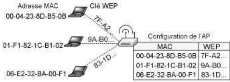
Figure 7.3 — Les clés WEP individuelles.
