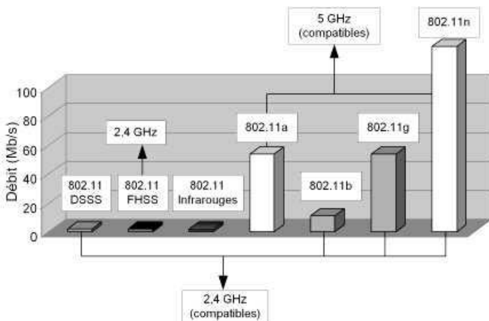
Figure 2.1 — Les couches physiques du WiFi : débit, fréquence et compatibilité.
