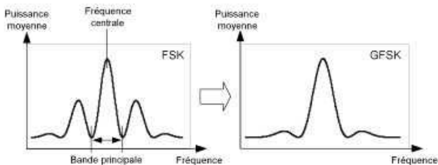
Figure 2.11 — Atténuation des fréquences harmoniques grâce au filtre Gaussien.
