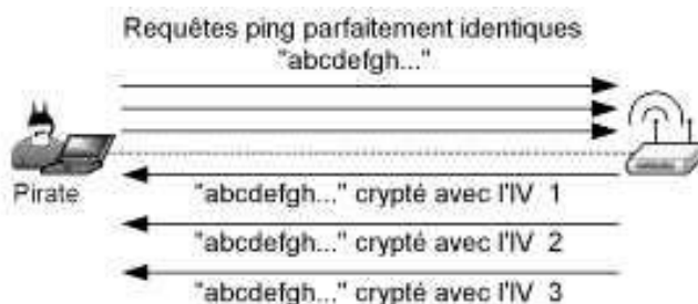
Figure 7.7 — Constitution d'un dictionnaire de décryptage grâce aux requêtes ping.
