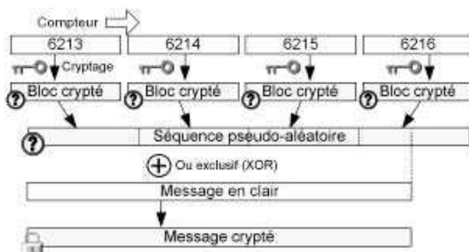
Figure 9.14 — Le Counter-Mode (mode compteur)
