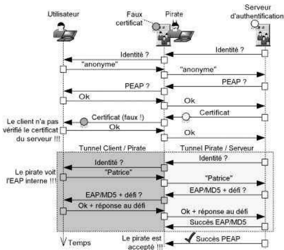
Figure 8.12 — Attaque MiM contre les authentifications reposant sur TLS.
