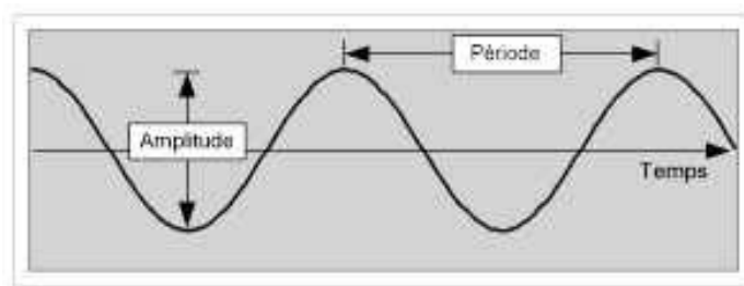
Figure 2.2 — Une onde et ses grandeurs physiques.
