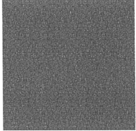
(d) 10 iterations
